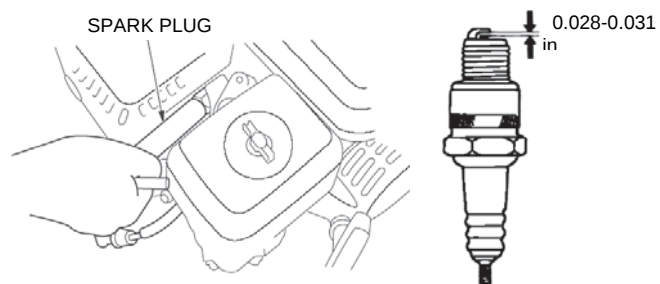
Figure 34 — Changer la bougie d'allumage
