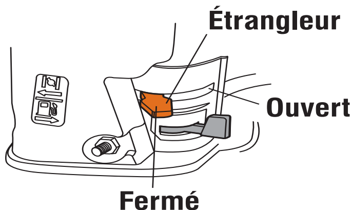
Figure 24 - Levier d'étrangleur
