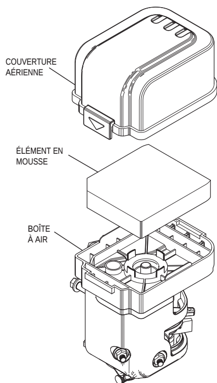
Figure 33 — Entretenir le filtre à air
