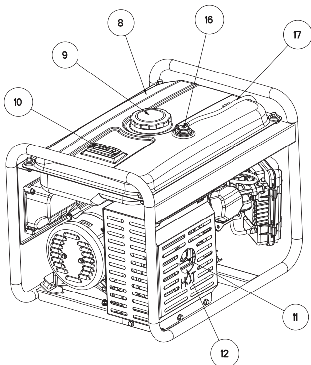
Figura 4 - Silenciador
